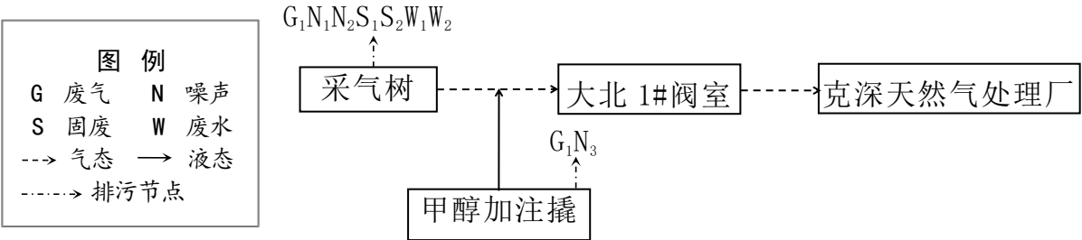
图 3.3-5 井场油气开采及集输工艺流程图
