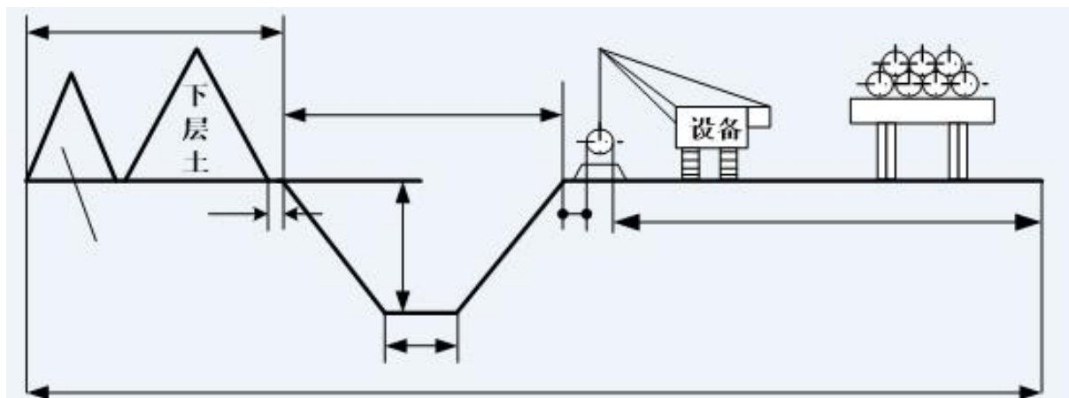
图 3.3-3 一般地段管道施工方式施工作业带断面示意图
