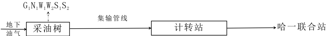
图 3.3-6 采油井场油气开采及集输工艺流程图
