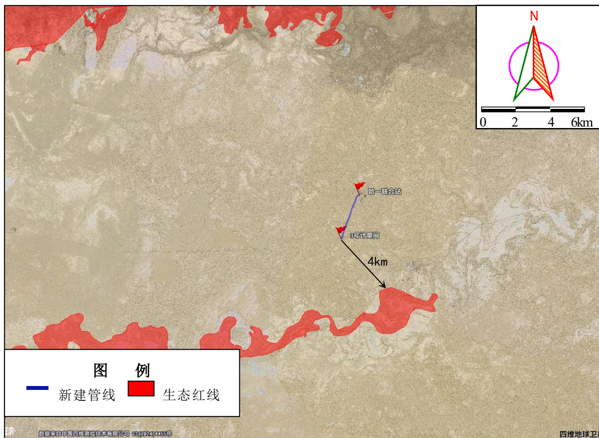
图 2.7-1 本项目管线方案施工图
