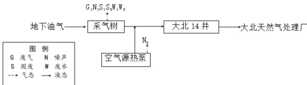
图 3.3-5 井场油气开采及集输工艺流程图
