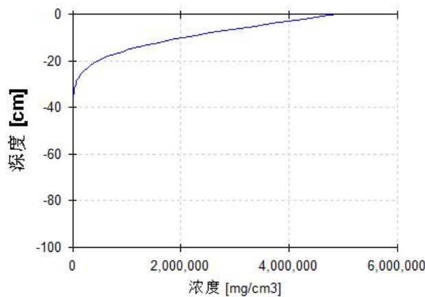
图 5.2-5 石油烃沿土壤垂向迁移情况
