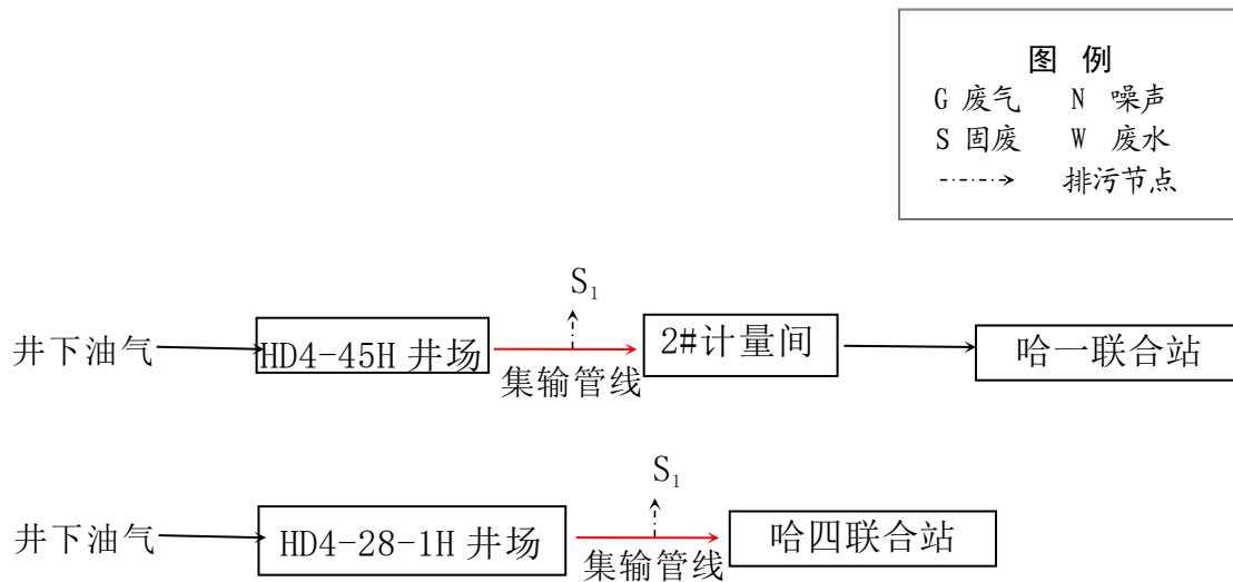
图 3.3-4 油气集输工艺流程图
