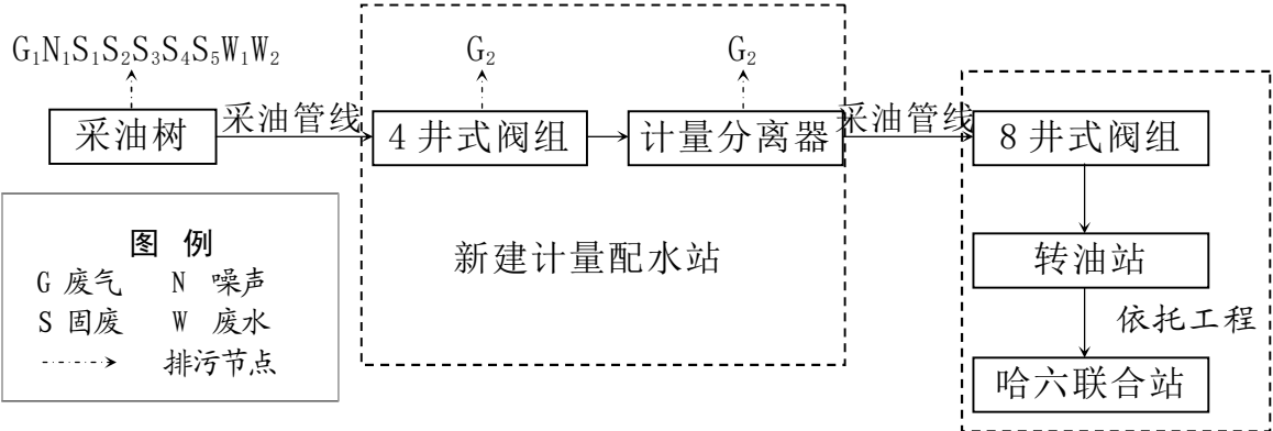
图 3.4-2 油气开采及集输工艺流程图
