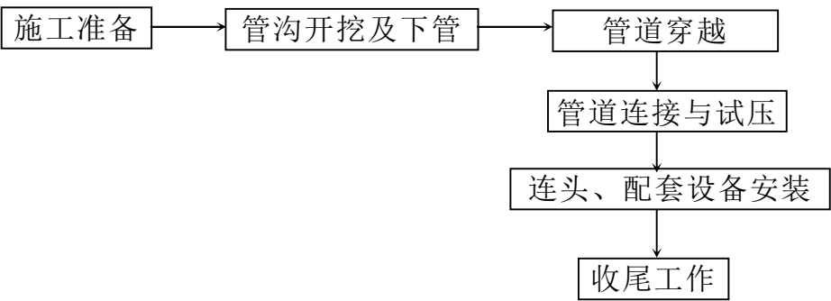
图3.4-1 施工方案工艺流程图
