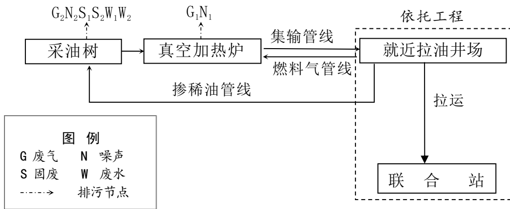
图 3.3-5 集输井场工艺流程图
