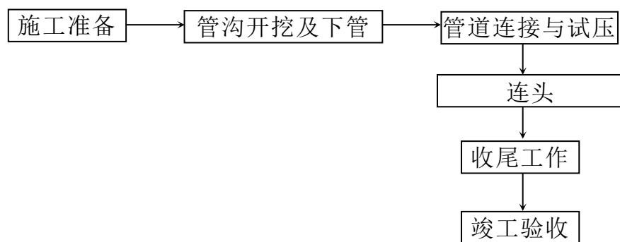
图3.3-3 施工阶段工艺流程图
