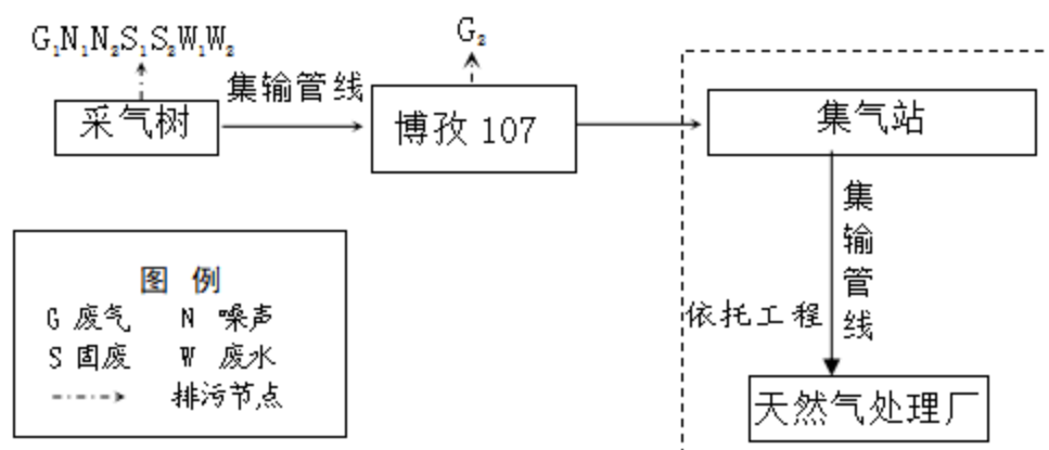
图 3.4-5 井场油气开采及集输工艺流程图
