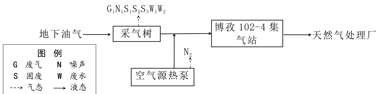
图 3.4-4 井场油气开采及集输工艺流程图
