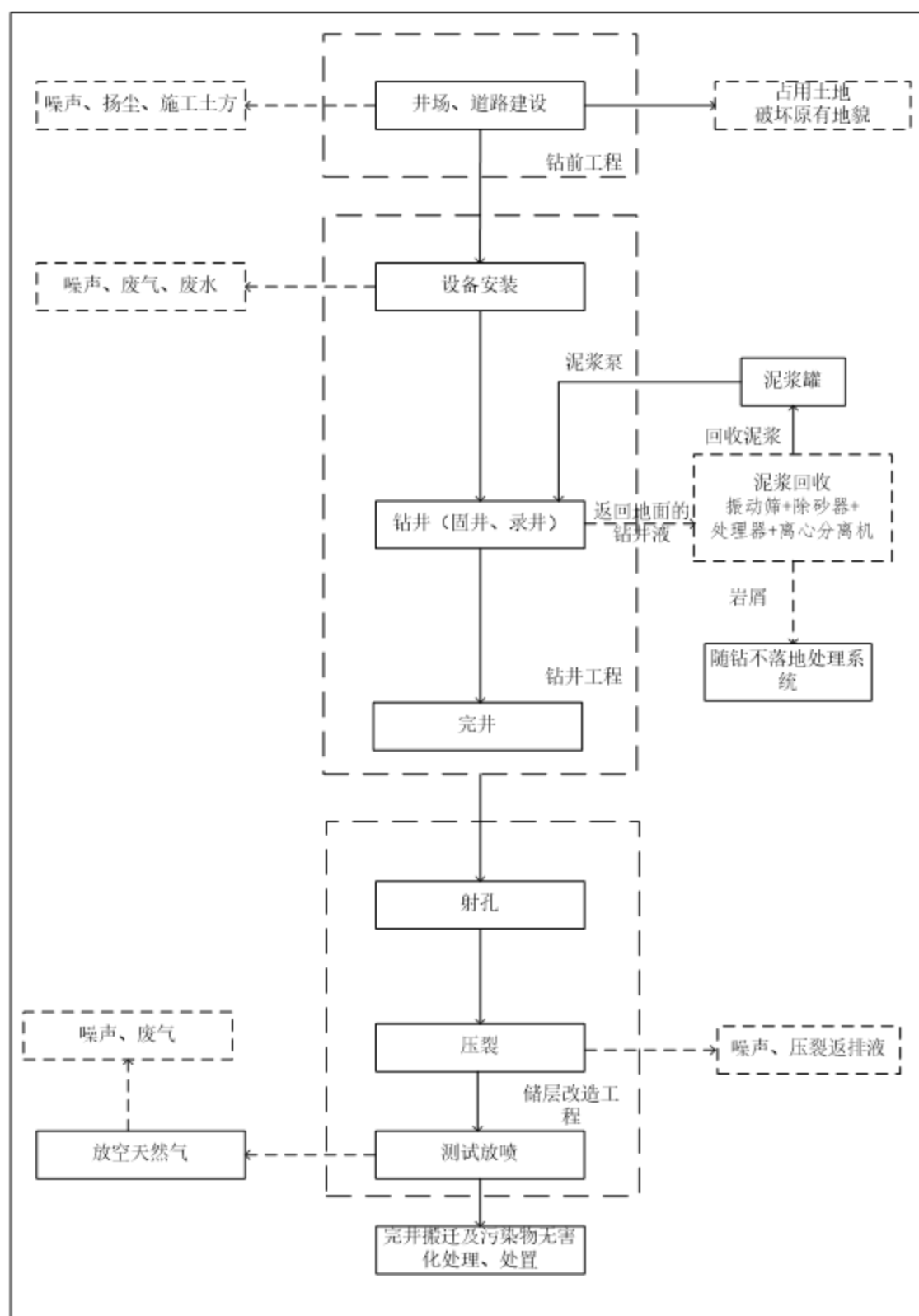
图 3.3-1 钻井工艺流程及污染物排放示意图
