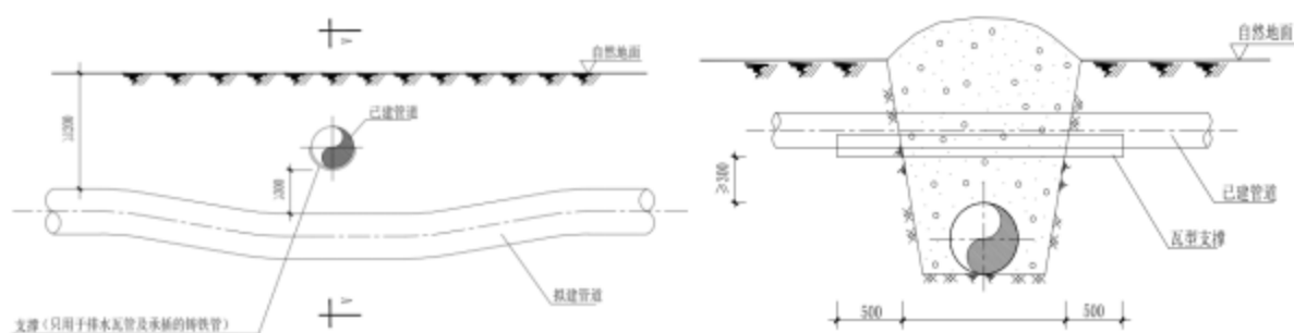
图 3.3-5 管道交叉施工作业示意图
