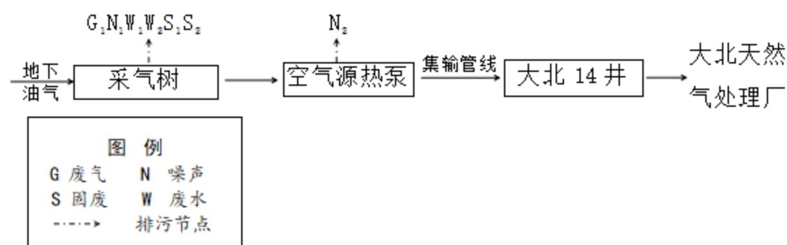
图 3.3-6 井场油气开采及集输工艺流程图
