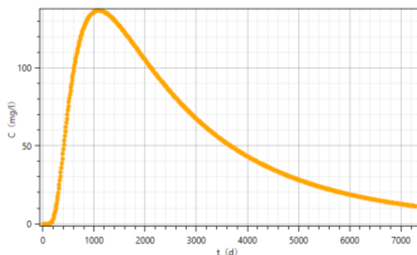
图5.2-7 非正常状况下，井场边界氯化物浓度变化曲线图
