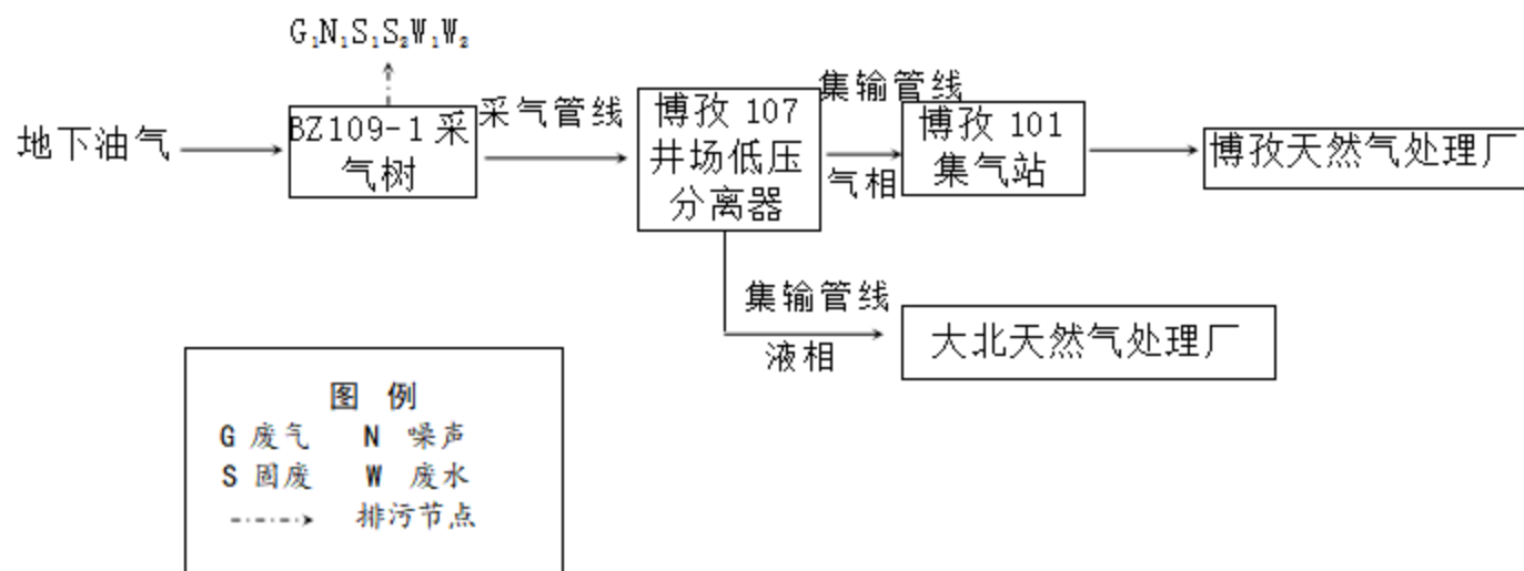
图 3.4-6 低压生产阶段油气开采及集输工艺流程图
