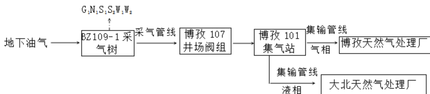
图 3.4-5 高压生产阶段油气开采及集输工艺流程图
