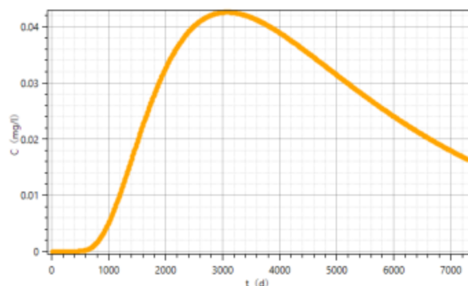
图5.2-5 非正常状况下，井场边界石油类浓度变化曲线图
