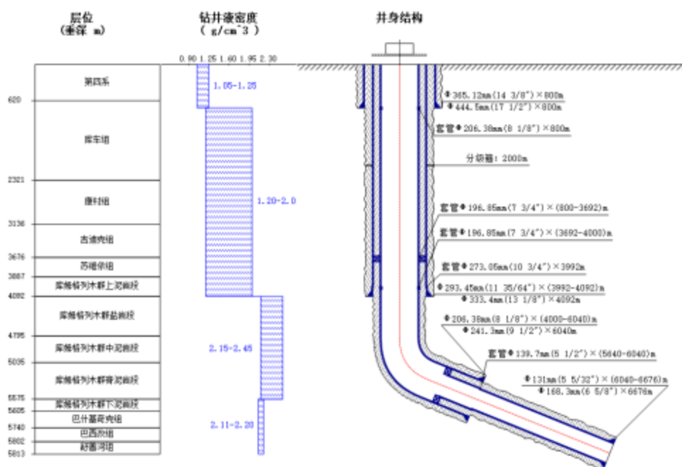
图 3.3-1 井身结构示意图。
