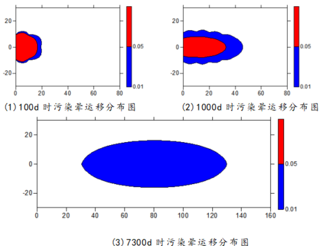
图 5.2-4 非正常状况下，石油类渗漏含水层影响范围图
