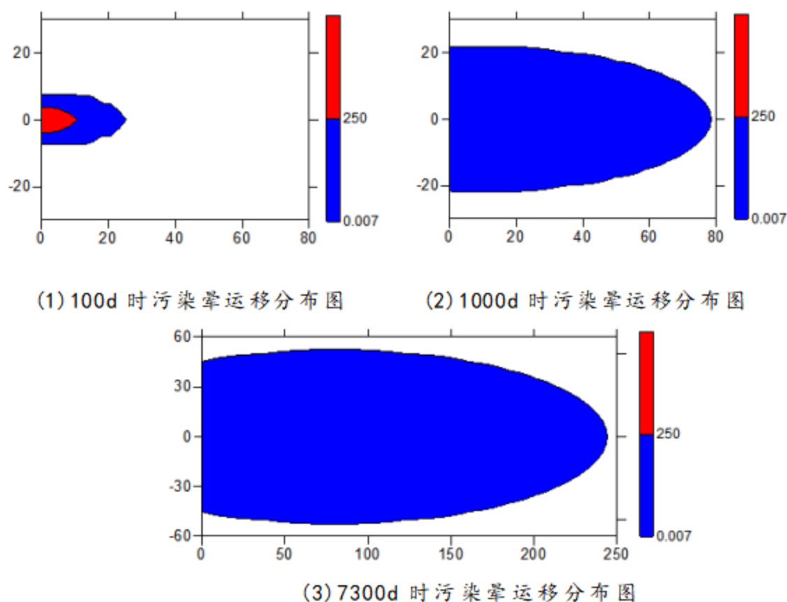
图 5.2-6 非正常状况下，氯化物渗漏含水层影响范围图
