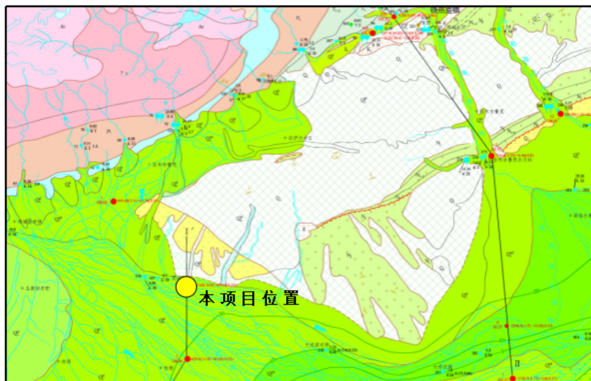
图 5.2-1 区域水文地质图
