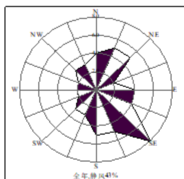
图 5.5-1 近 20 年风频玫瑰图
