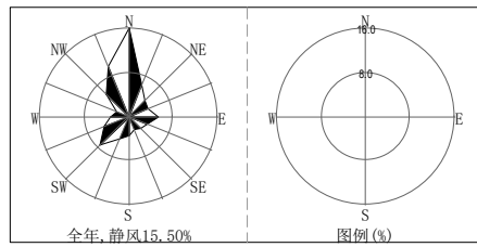
图 5.2-1 区域近 20 年风频玫瑰图
