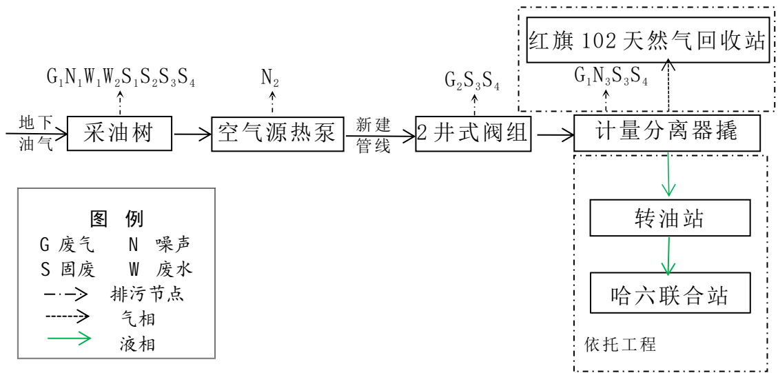
图 3.4-4 井场油气开采及集输工艺流程图
