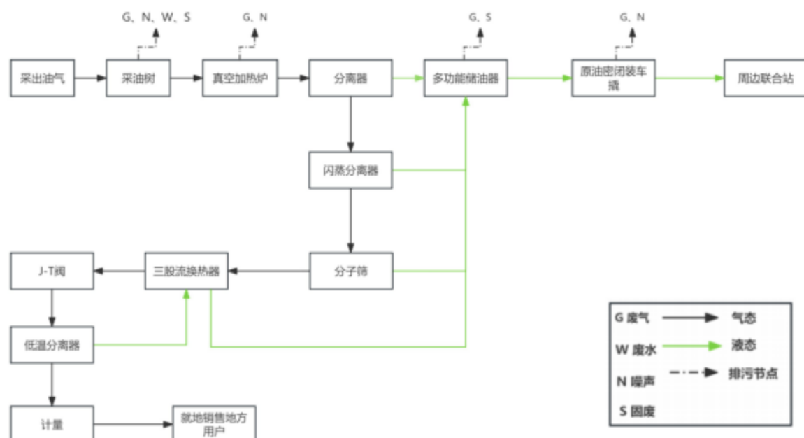
图 3.3-6 拉油井场油气开采及集输工艺流程图
