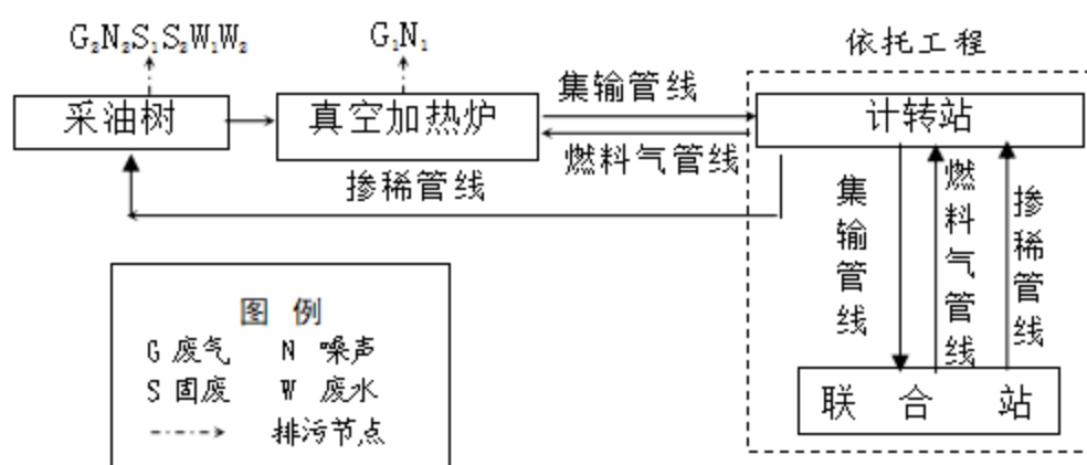
图 3.3-6 管输井场油气开采及集输工艺流程图
