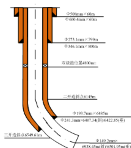
(3) 水平井井身结构
