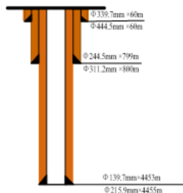
(2) 油井二级井身结构
