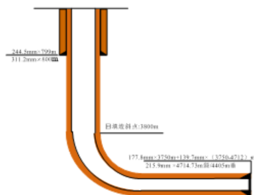
(1) 水平井井身结构
