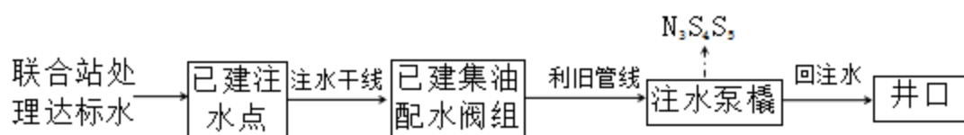
图 3.5-6 注水工艺流程图
