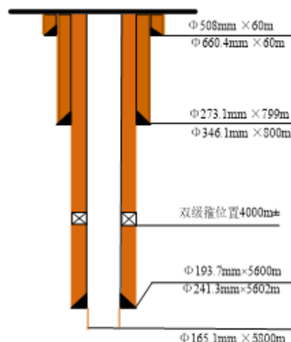
(4) 新三级井身结构-直井
