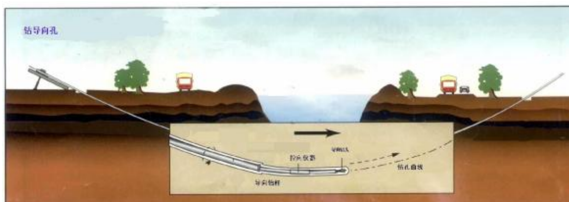
图3.4-2 钻导向孔示意图
