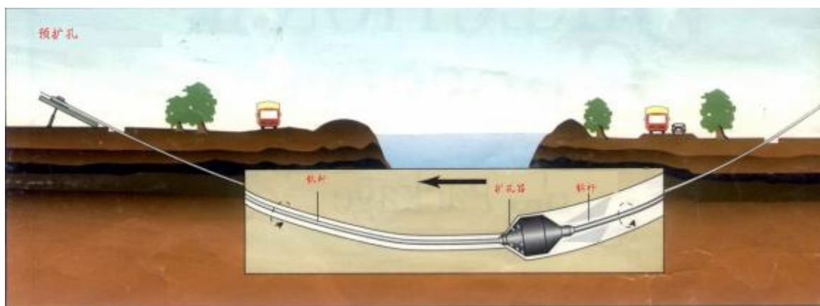
图3.4-3 预扩孔示意图
