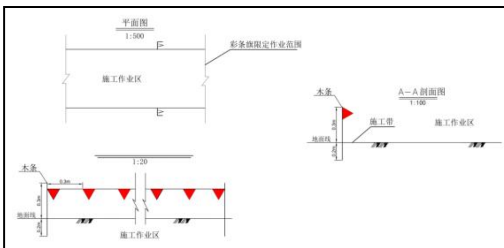
图 6.1-2 限行彩条旗典型措施设计图
