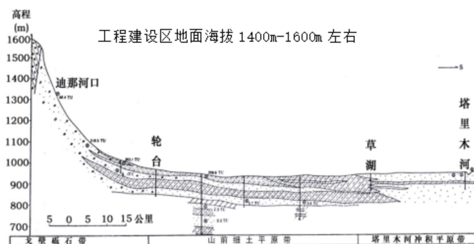
图 5.2-1 迪那河洪积扇地质结构剖面示意
