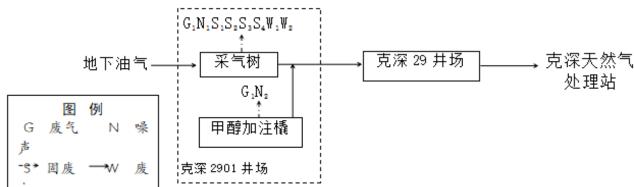
图 3.4-5 拟建工程油气开采及集输工艺流程图
